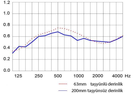
EN ISO 354 ses yutma katsayısı ölçümü
